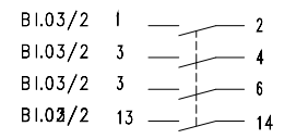
Hauptschütz
